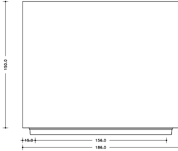
SEZIONE LONGITUDINALE
