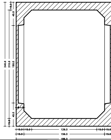
SEZIONE TRASVERSALE
