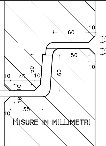
SEZIONE TRASVERSALE
